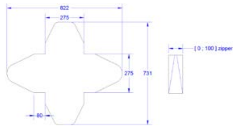
Schéma de principe du pod fourni :
