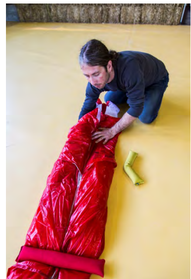
Fig. 102 Posez une moitié sur l'autre
